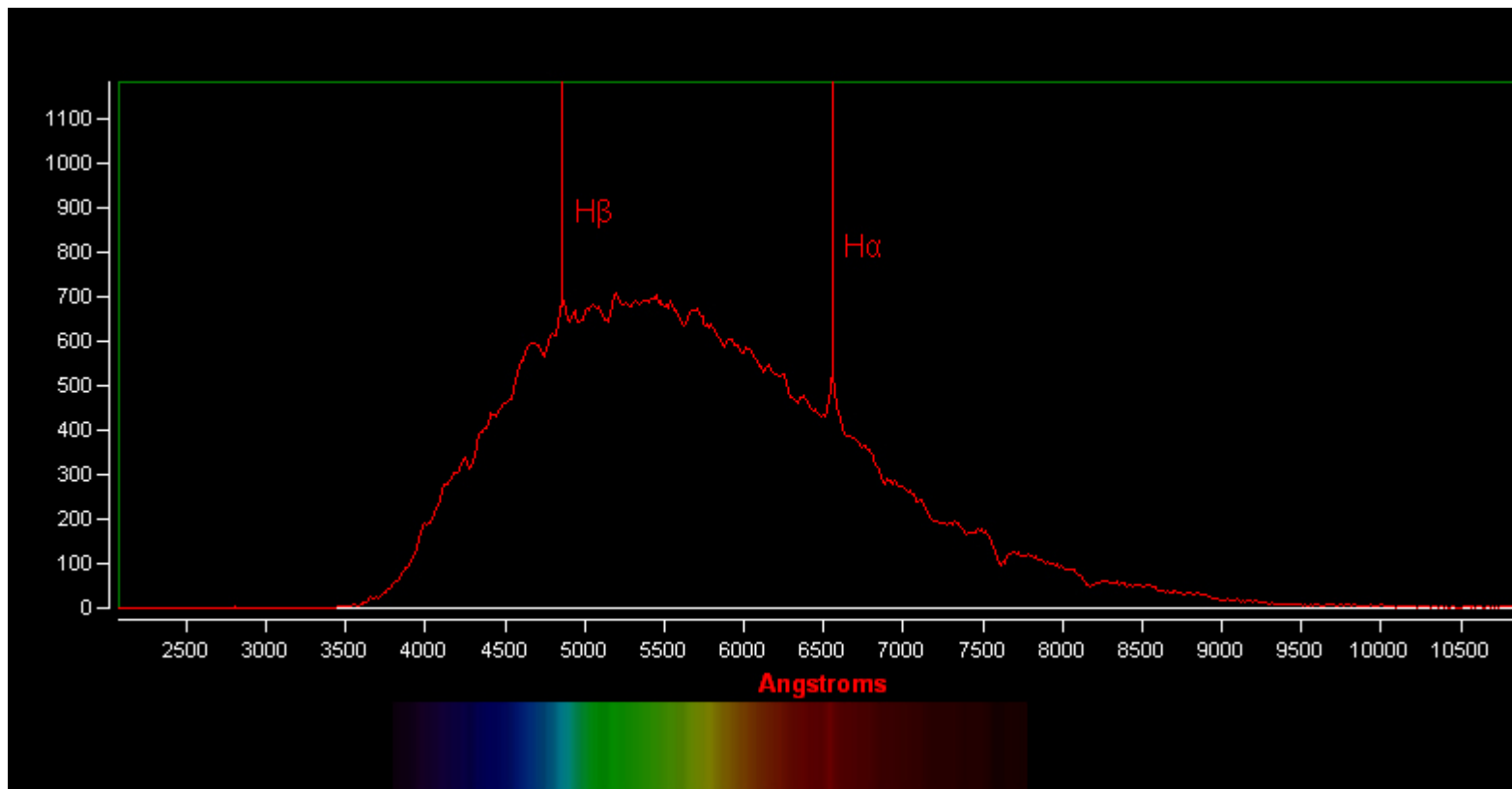
Spettro del 18/08/2013: il grafico mostra una graduale ripresa dell'emissione Hbeta mentre resta invariata quella Halpha.
